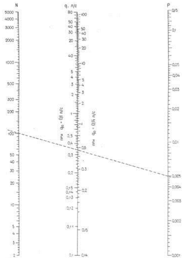
Черт. 1. Номограмма для определения секундных расходов воды q при q_0 = 0,1 и 0,14 л/с и P \in 0,15
